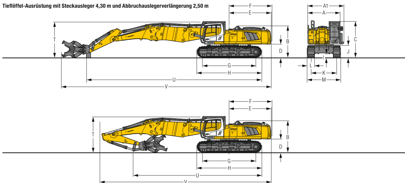
Tieflöffel-Ausrüstung mit Steckausleger 4,30 m und Abbruchslegerverlängerung 2,50 m
